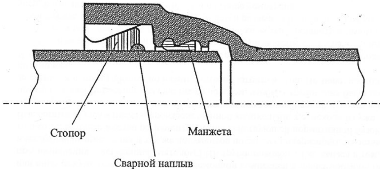
Рисунок 7.3 – Разрез раструбно-замкового соединения
