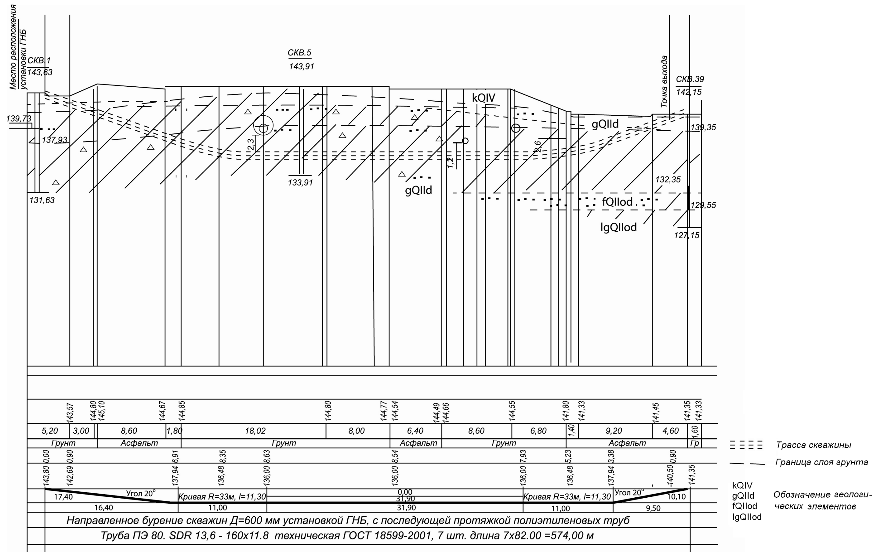
Рисунок 7.1 – Пример построения продольного профиля трассы скважины ГНБ
