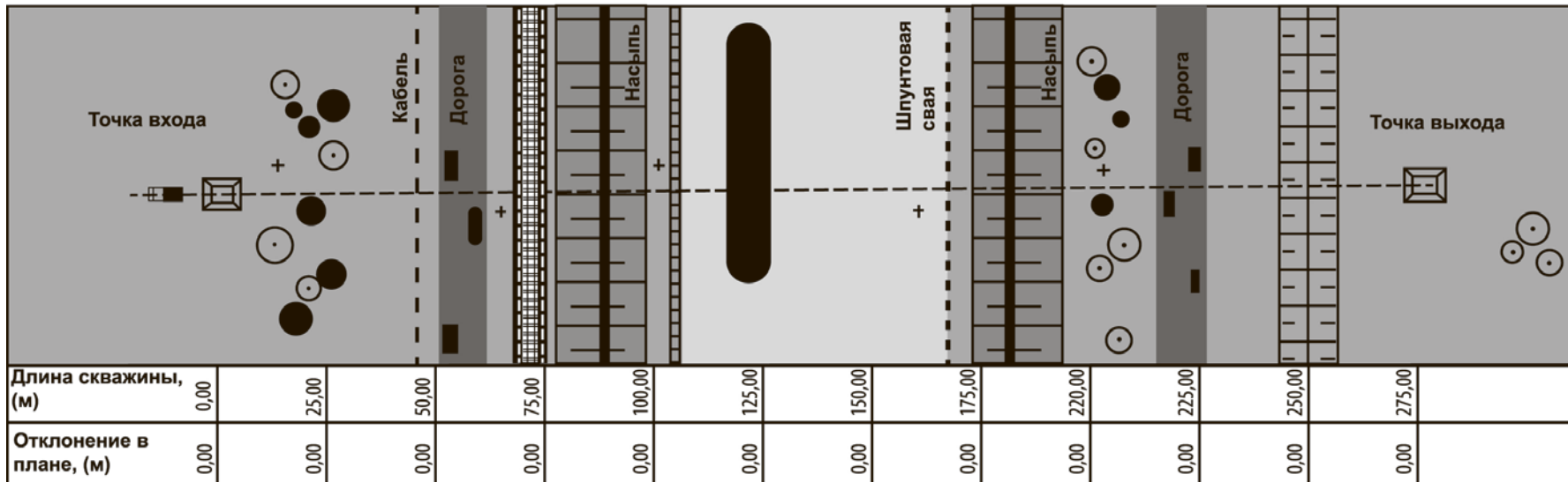
Рисунок А.1– Продольный профиль и план закрытого подземного перехода, сооружаемого методом ГНБ
