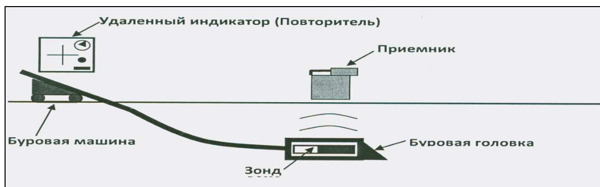
Рисунок ВГ.2 – Схема действия электромагнитной системы подземной локации
