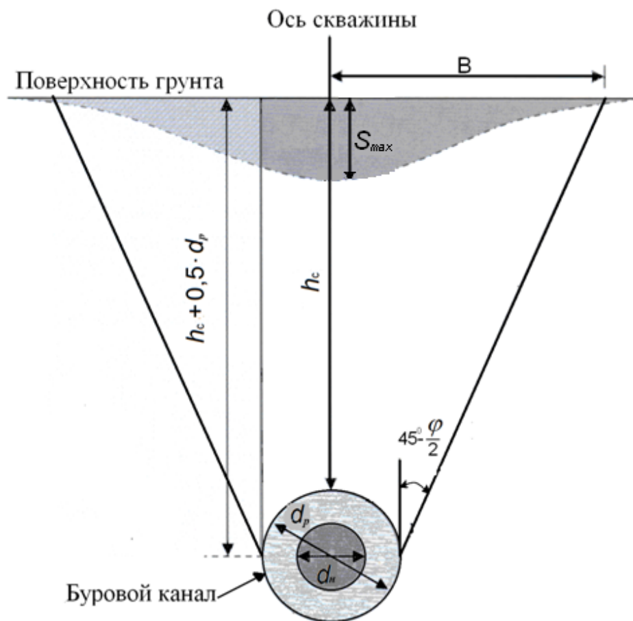
Рисунок 7.2 – Распределение осадок поверхности для скважин ГНБ
