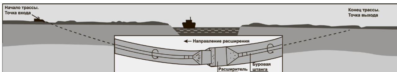
Рисунок 8.4—Расширение скважины
