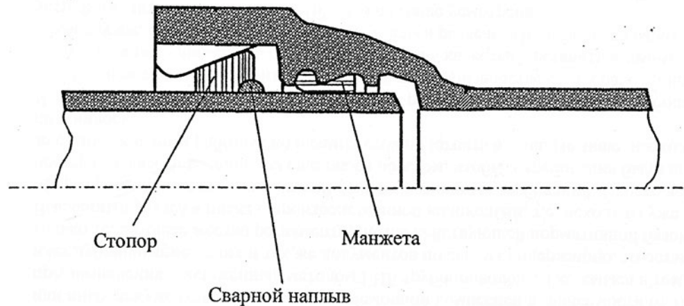
Рисунок 7.3 – Разрез раструбно-замкового соединения
