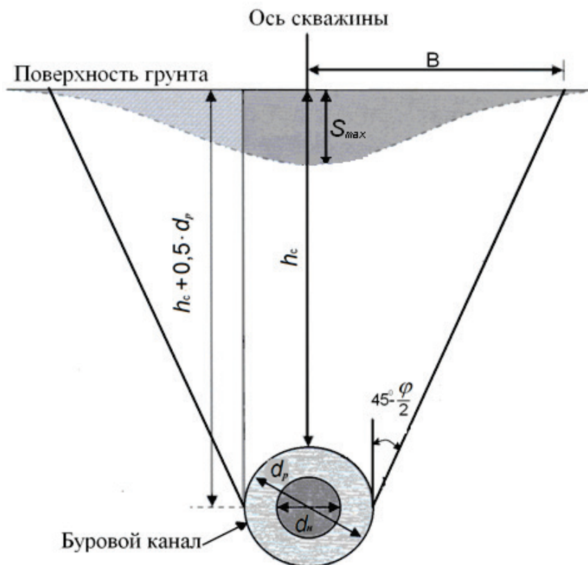
Рисунок 7.2 – Распределение осадок поверхности для скважин ГНБ
