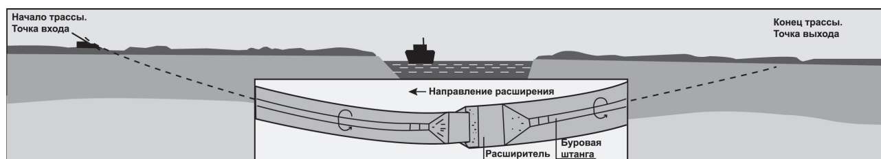
Рисунок 8.4 – Расширение скважины
